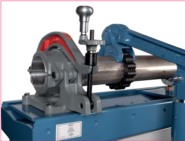
Фрикционные тиски и трубные ключи
