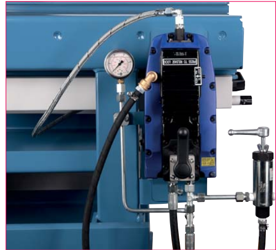
Силовая гидравлическая установка с ремонтным комплектом
